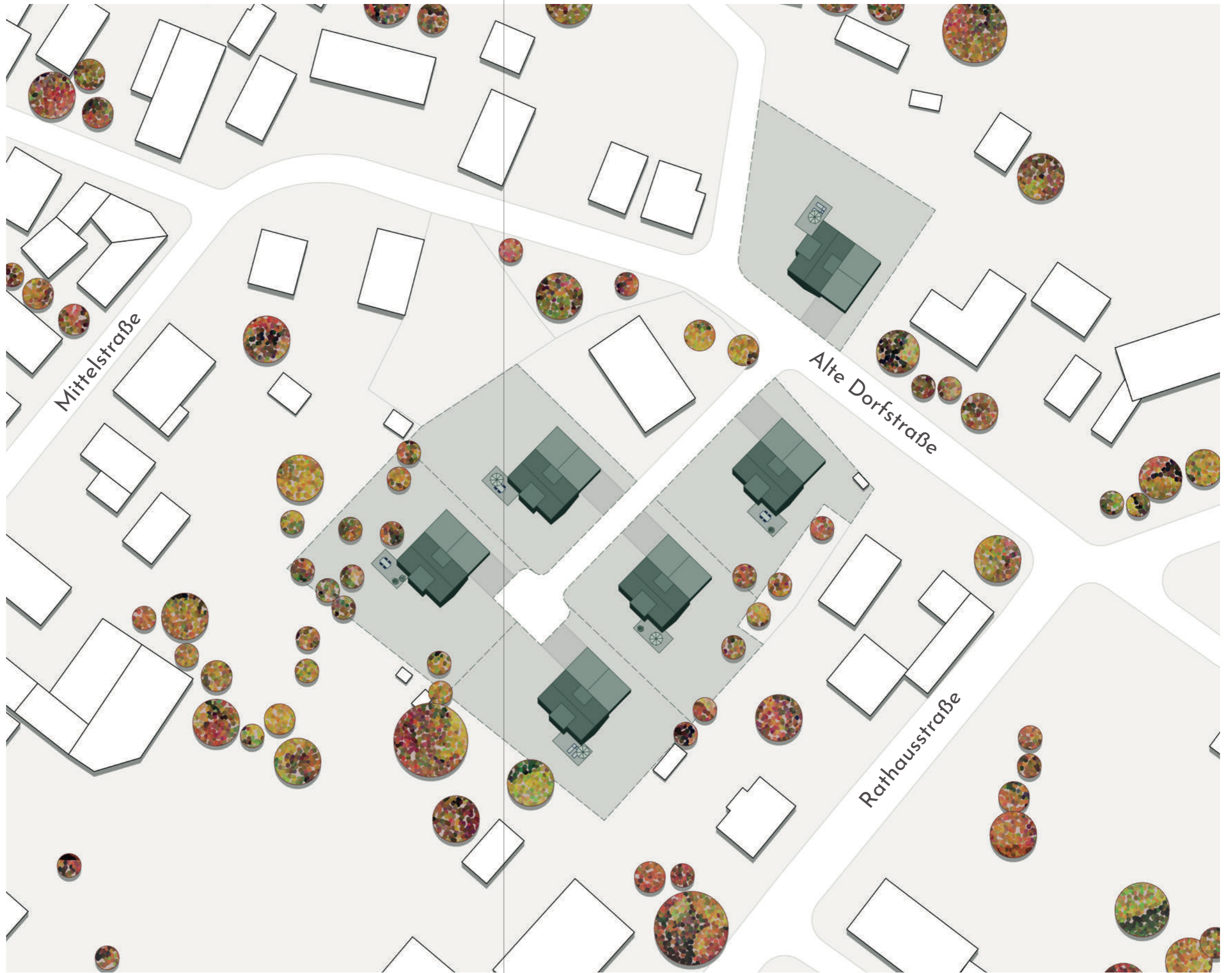
Übersichtslageplan
